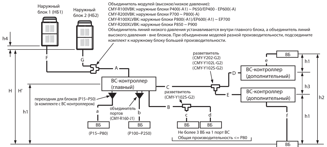
НБ - наружный блок, ВБ - внутренний блок, ВС - ВС-контроллер
