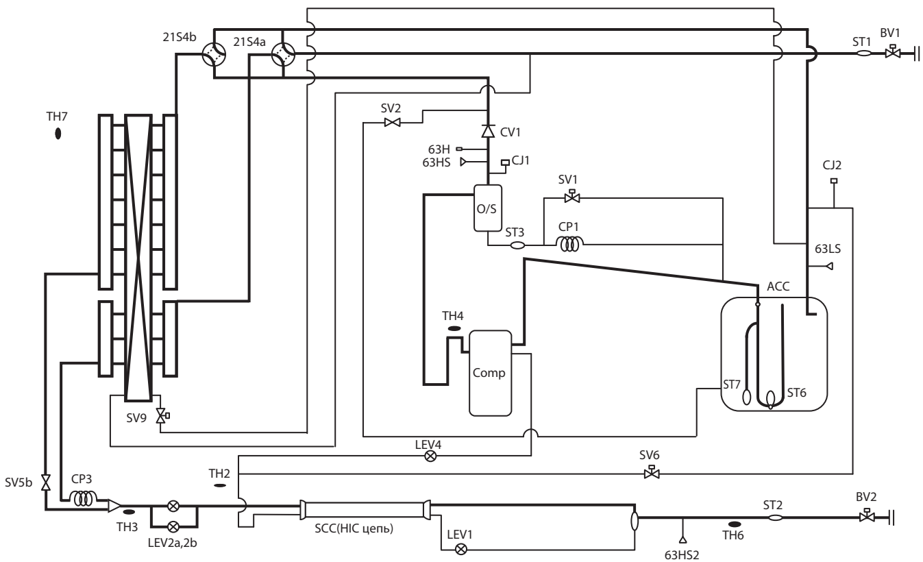
(4) PUHY-HP200, HP250YHM-A
