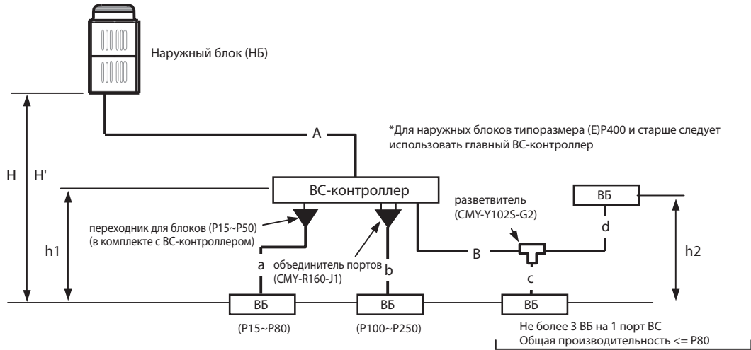
НБ - наружный блок, ВБ - внутренний блок, ВС - ВС-контроллер
