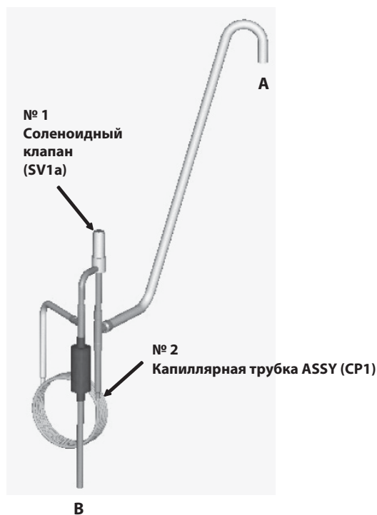
Соленоидный клапан ASSY
