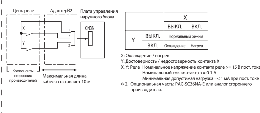
(3) CN3N
